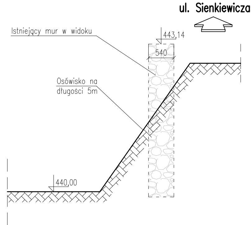
STAN ISTNIEJĄCY PRZEKRÓJ POPRZECZNY A-A skala 1:50
