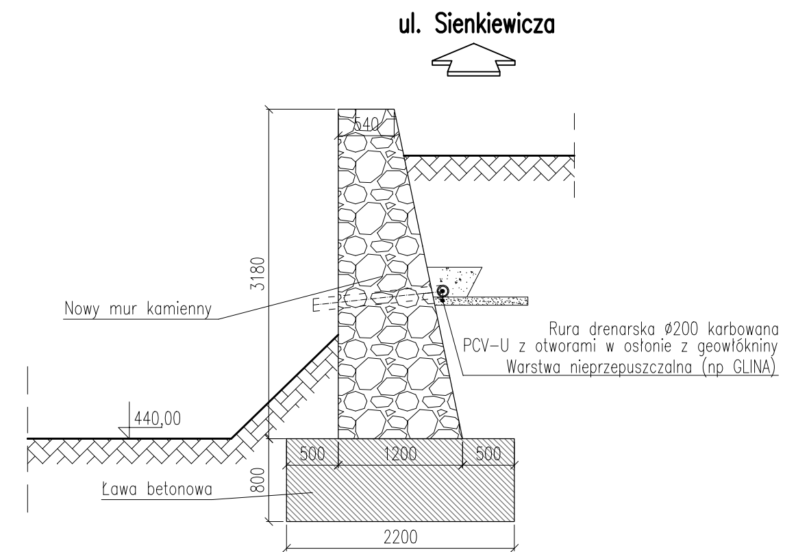
STAN PROJEKTOWY PRZEKRÓJ POPRZECZNY A-A skala 1:50
