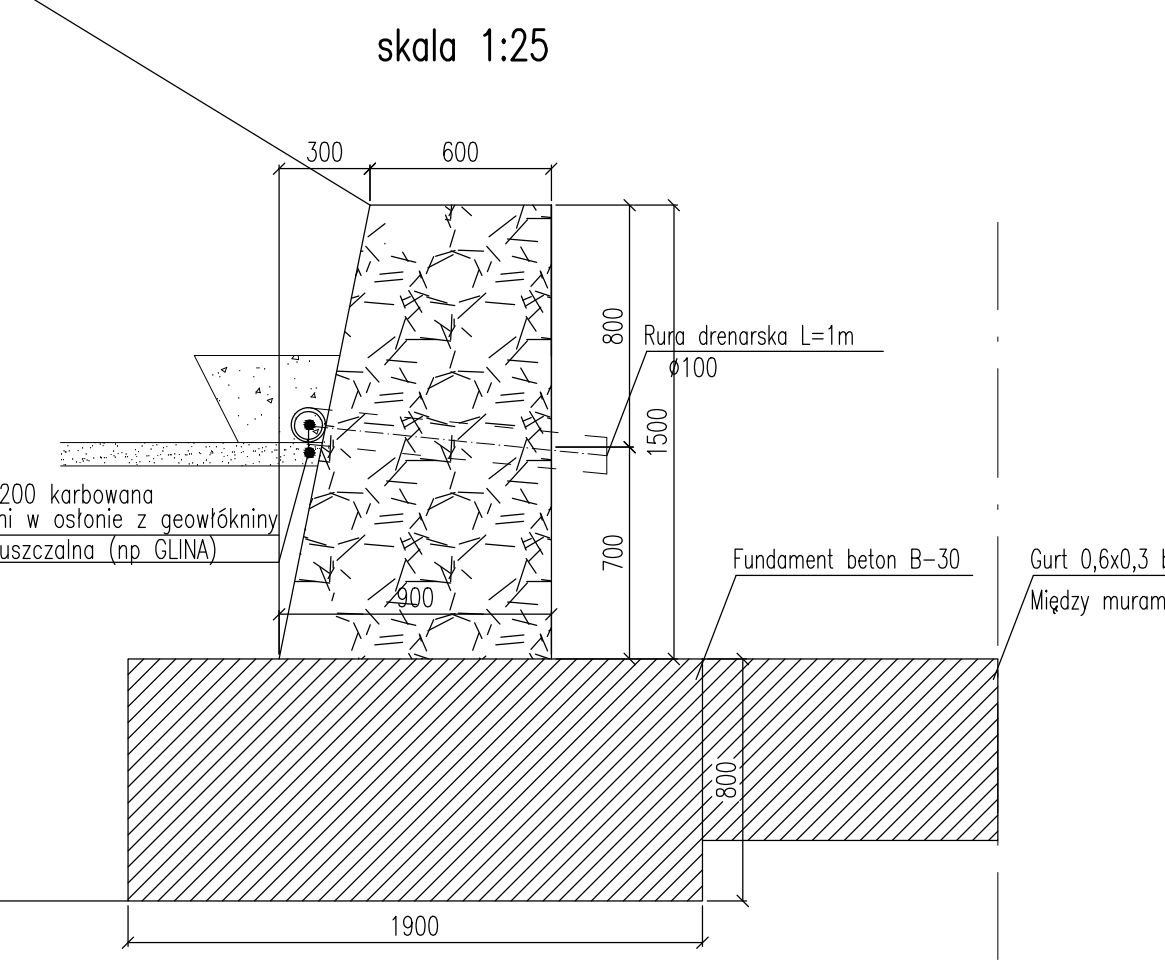
R1 – BUDOWA MURÓW KAMIENNYCH H DO 1,5 m Z GURTAMI PRZEKRÓJ POPRZECZNY CHARAKTERYSTYCZNY MURU skala 1:25
