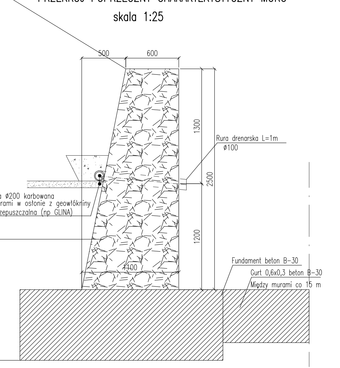
R2 – BUDOWA MURÓW KAMIENNYCH H DO 2,5 m Z GURTAMI PRZEKRÓJ POPRZECZNY CHARAKTERYSTYCZNY MURU skala 1:25
