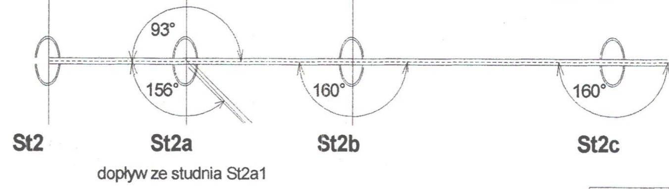
St2a studnia kaskadowa
